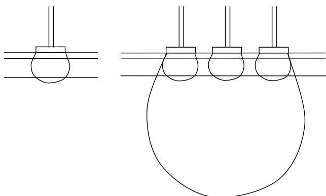
Bulbe des contraintes d'une charge ponctuelle isolée
