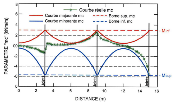
Terme correctif représentant l'interaction entre les inclusions rigides et les joints du dallage.
