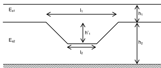
Exemple d'hétérogénéité : zone d'ancien bras mort remblayée
