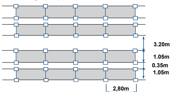
Exemple de rayonnages classiques dos à dos
